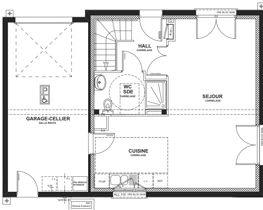
PLAN RDC
