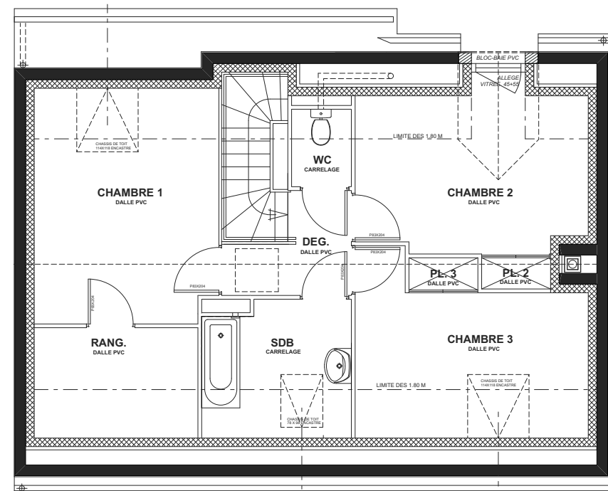
PLAN ETAGE
