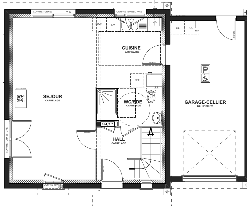
PLAN RDC
