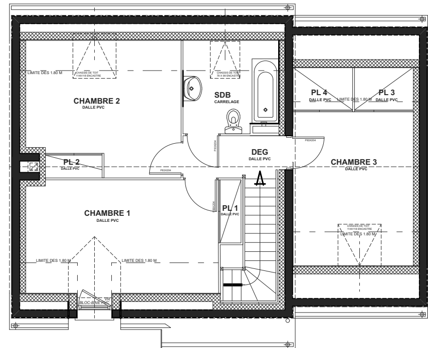
PLAN ETAGE
