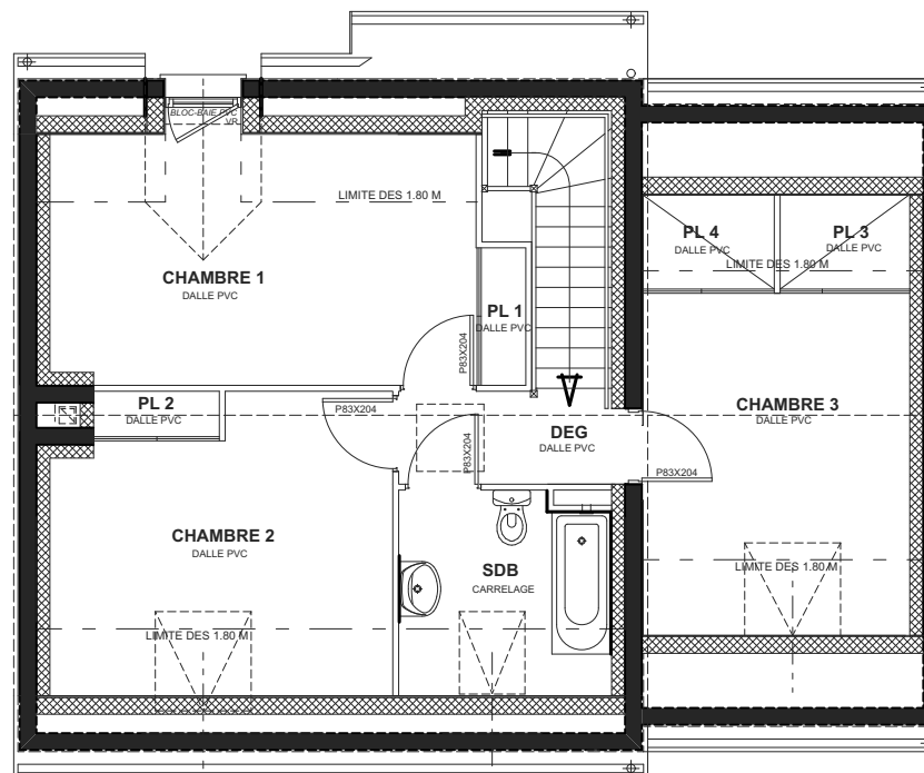
PLAN ETAGE
